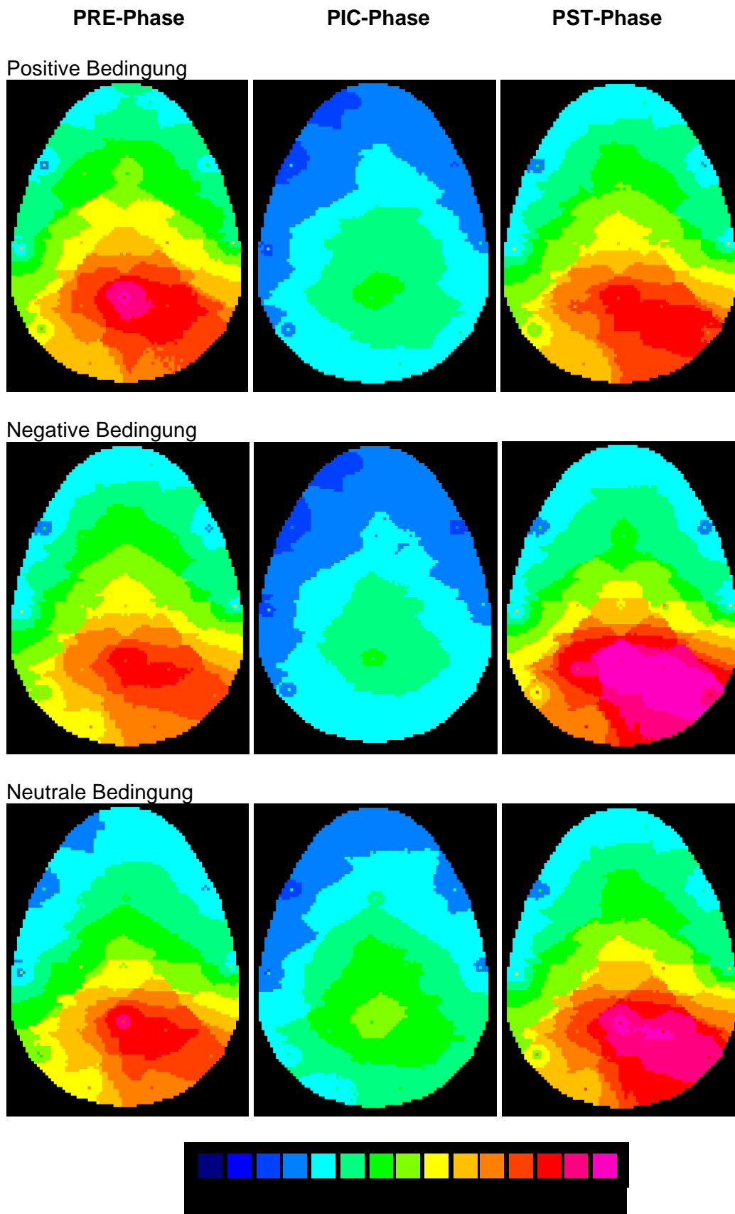
Abbildung 9: EEG-Alpha-Band der nicht-logarithmierten Rohdaten in der positiven, negativen und neutralen Bedingung vor (PRE), während (PIC) und nach (PST) der Bilddarbietung. Aus technischen Gründen ist das Frequenzband zwischen 7.8 Hz und 13 Hz dargestellt.
